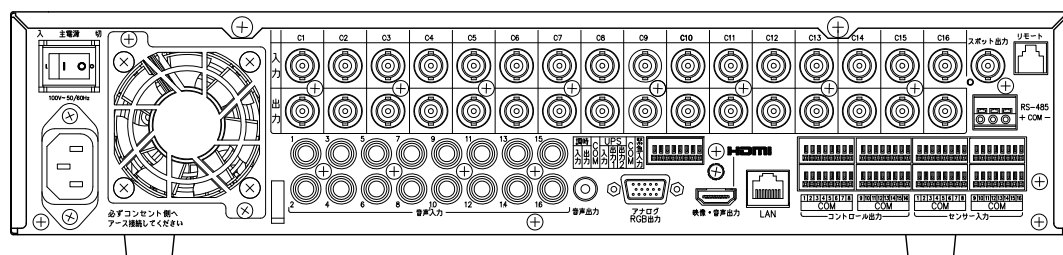
背面図
