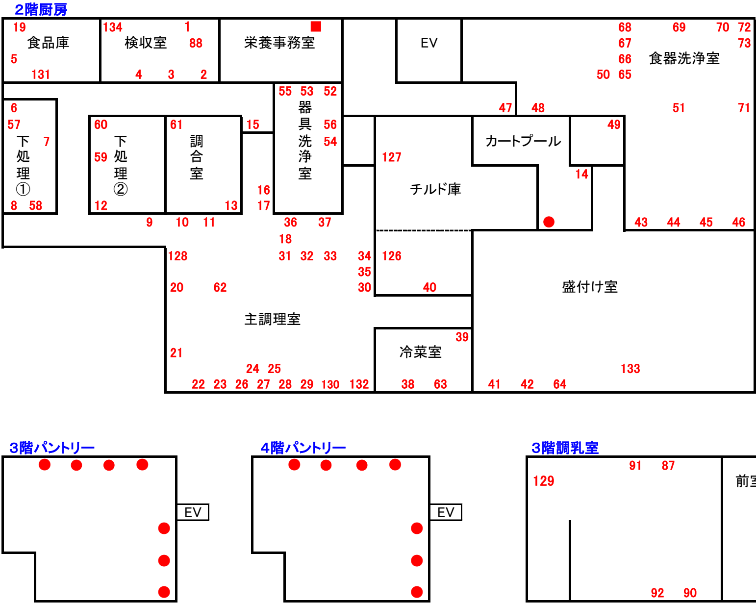
【厨房機器類配置図】
